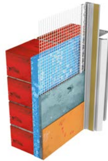
646900 Kombi Laibungsprofil mit Steglippe und Gewebe
